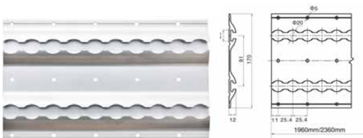
Rotaia Verticale Doppia
