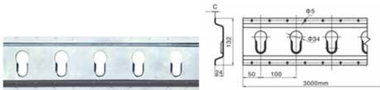
Rif. B9004 Profilo per barra appendiabiti Acciaio zincato , spessore mm 1,5, Lunghezza mm 3000
